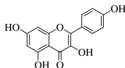
Kaempferol (2)
